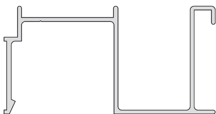
3005 / 20 Guía p/ cortina 428 grs / mt. 14 barras de 6.050 mm.
