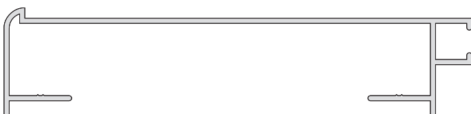
3005 / 10 Marco aireador 437 grs / mt. 12 barras de 6.050 mm.
