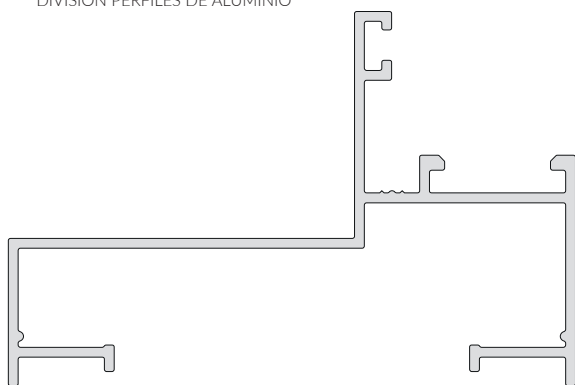
3050 / 176 Marco 75 715 grs / mt. 4 barras 6.150
