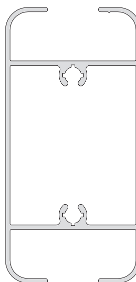
3050 / 67 Travesaño puerta vidrio simple 886 grs / mt. 6 barras de 6.050 mm.
