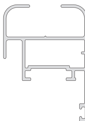
3050 / 62 Hoja ventana batiente vidrio simple 605 grs / mt. 4 barras de 6.050 mm.
