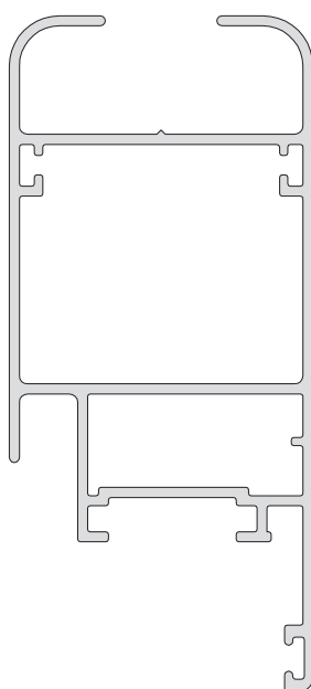
3050 / 66 Hoja puerta vidrio simple 945 grs / mt. 4 barras de 6.050 mm.
