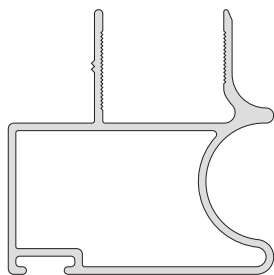
3034 / 01 Frente placard 416 grs / mt. 12 barras de 5.200 mm.
