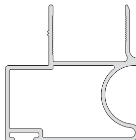
3034 / 14 Frente placard 413 grs / mt. 12 barras de 5.200 mm.
