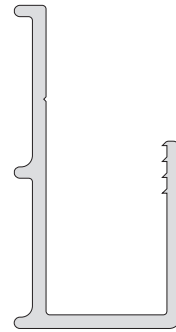
3060/14 437 g/m 12 barras de 6.050 mm.
