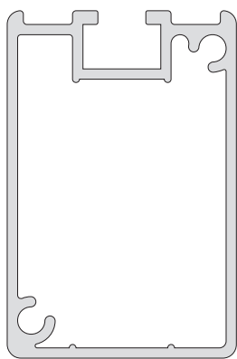
3060/02 830 g/m 6 barras de 6.050 mm.
